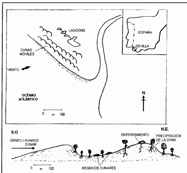
Fig. 4. Movimiento de dunas en el Parque Nacional de Doñana, observando la sucesiva lenta migración sobre el pinar. (Adaptado de Carter, 1995).
