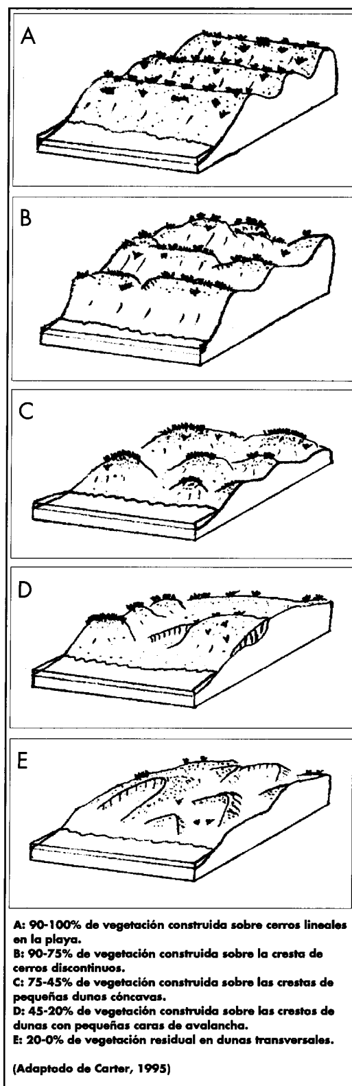
Fig. 2. Clasificación de dunas costeras basadas en la proporción de cobertura vegetal (según descripciones dadas por Short y Hesp, 1982).
