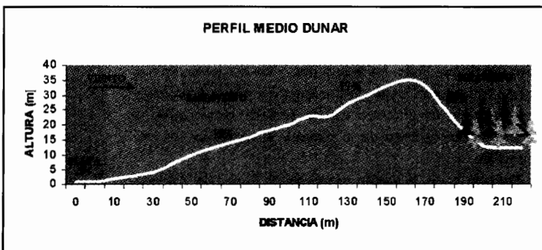
Fig. 10. Perfil topográfico "medio" de la Duna de Valdevaqueros,
