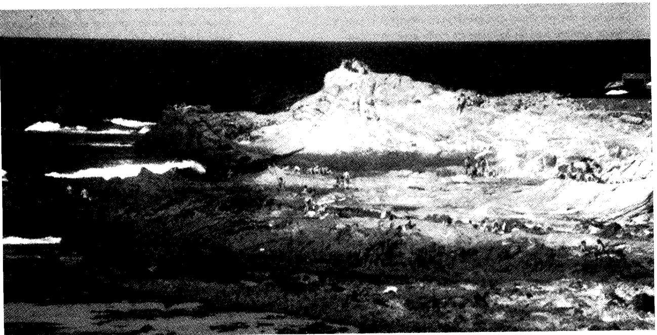
Figura 9. Uso del entorno rocoso del charco de Las Palomas (Aruacas, norte de Gran Canaria).
