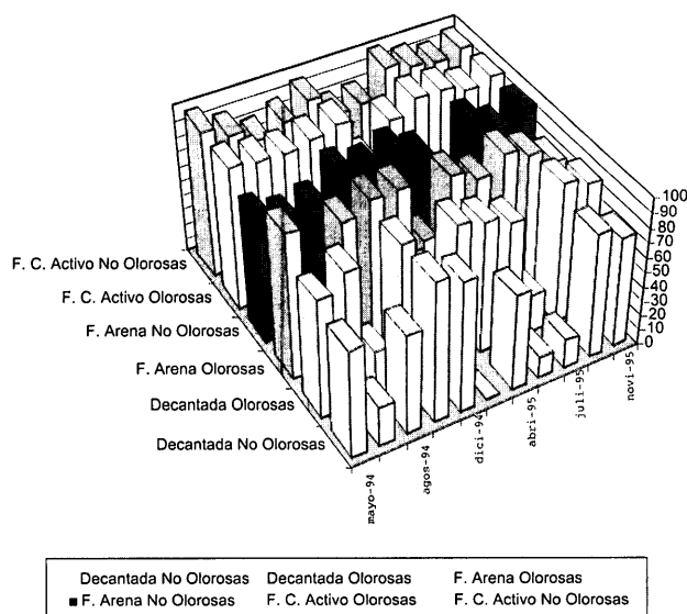
Gráfico 7. Eficacia de cada fase del proceso sobre algas olorosas y no olorosas.
