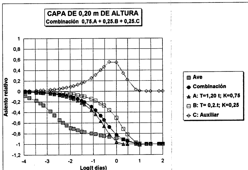
Fig. 5. Ejemplos de consolidación de dos capas de altura distinta.
