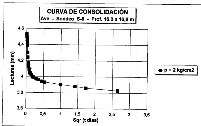
Fig. 1. Ejemplo de una curva de consolidación.
