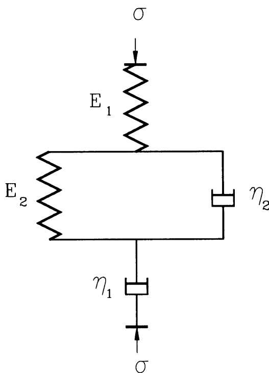
Fig. 2. Modelo viscoelástico de Burgers.
