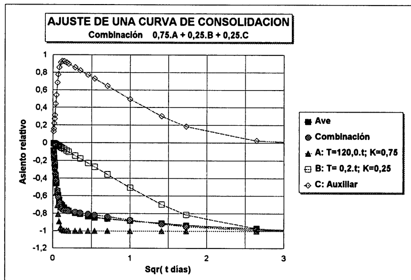
Fig. 4. Ajuste de las curvas de consolidación de la Fig. 1.
