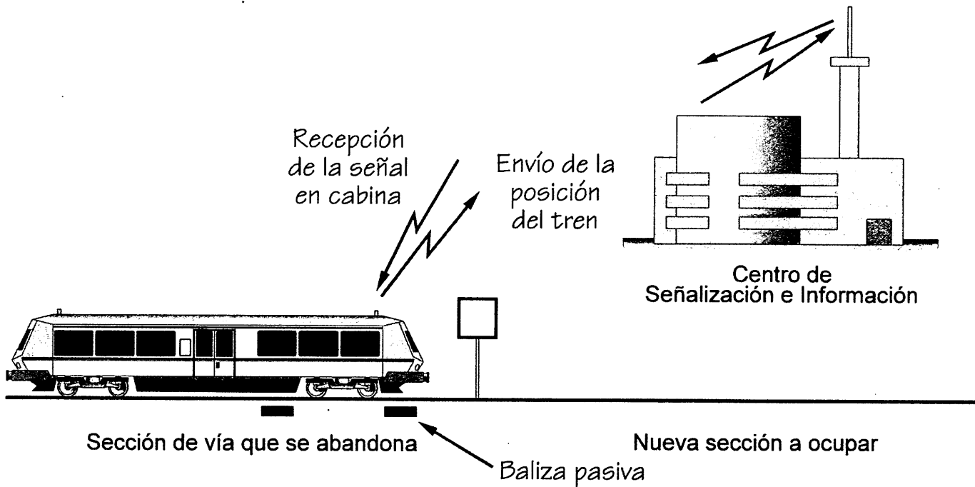
Figura 9. Bloqueo por radio.
