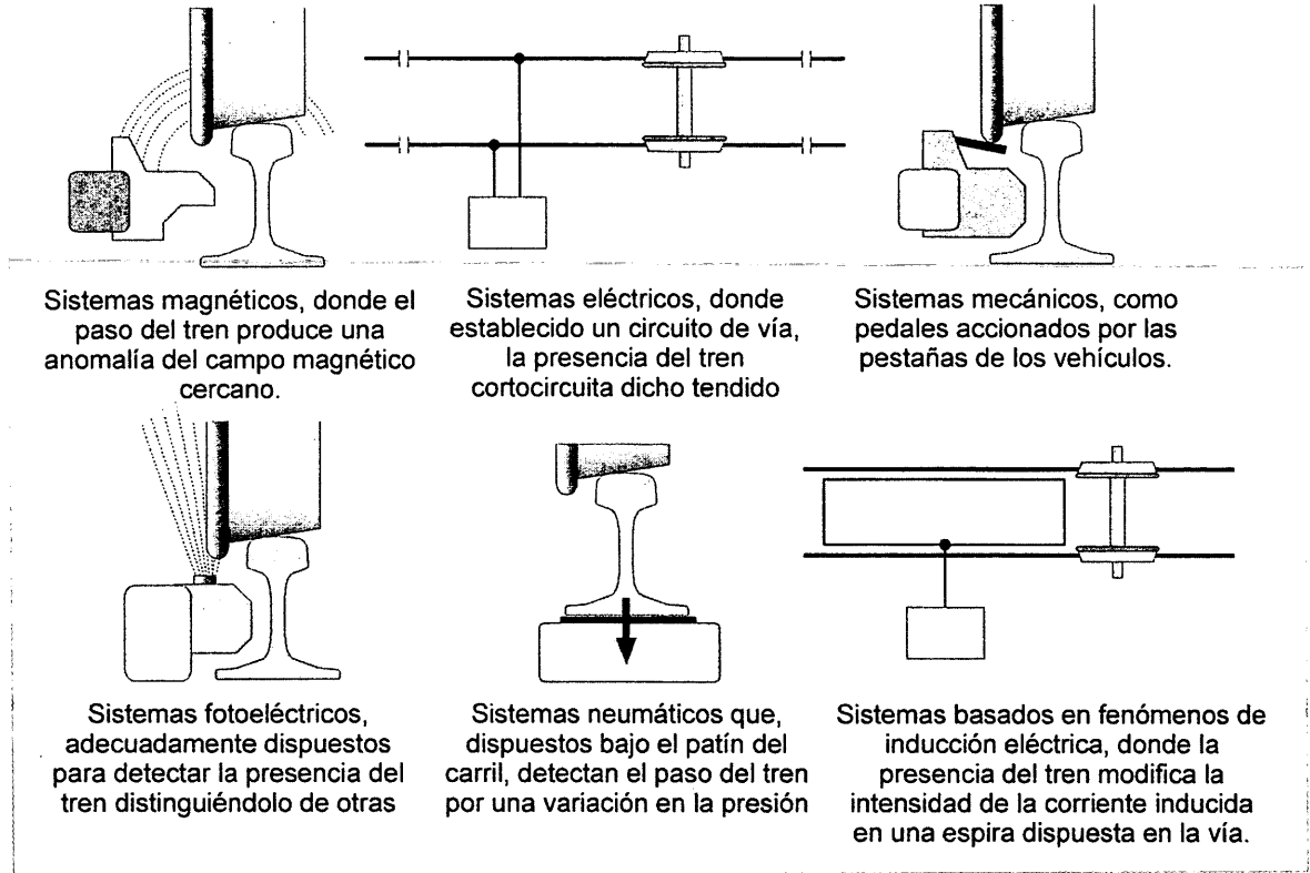
CUADRO 2. Sistemas de detección de trenes para protección de pasos a nivel
