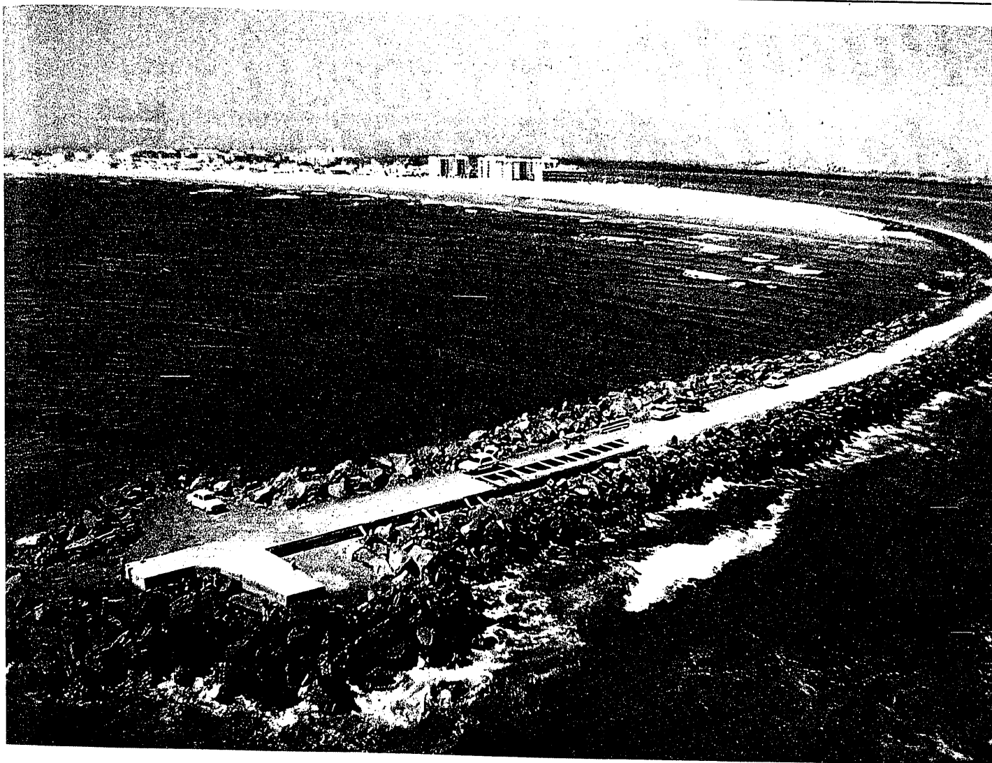
Figura n.º 8. Vista aérea del dique de Punta Umbria.
