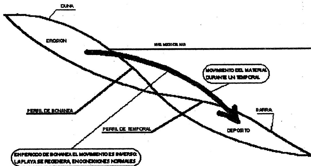
Figura n.º 5. Movimiento del perfil de playa durante un temporal.
