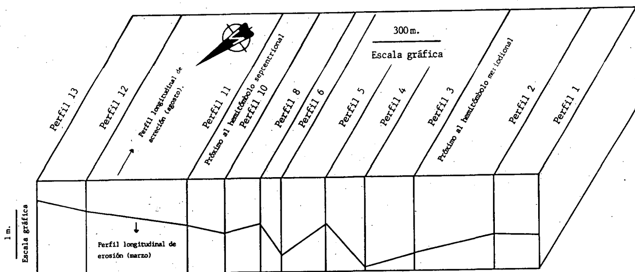
Figura 3. — Movimientos longitudinales en la playa de Las Canteras (Las Palmas).
