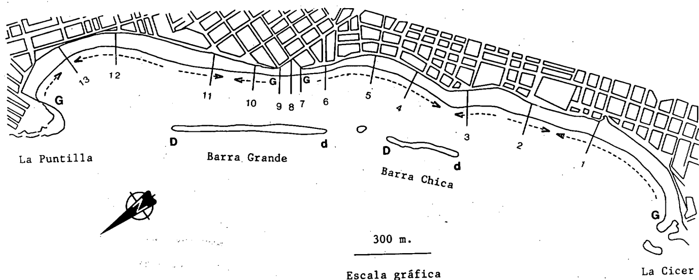
Figura 2.—Playa de Las Canteras (Las Palmas): Localización de los perfiles transversales en seguimiento y diagrama de transportes intermareales, según los valores del parámetro granulométrico Q_2 , con oleaje del alisio.
