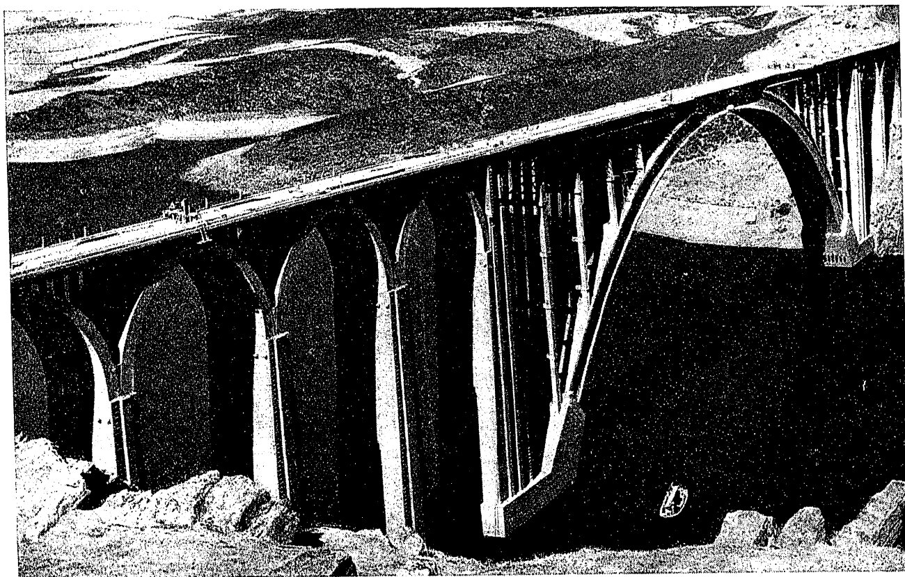
Viaducto del Esla. (Martín Gil, Jacobson, Peña Bocuf, Torroja y Salazar.)
