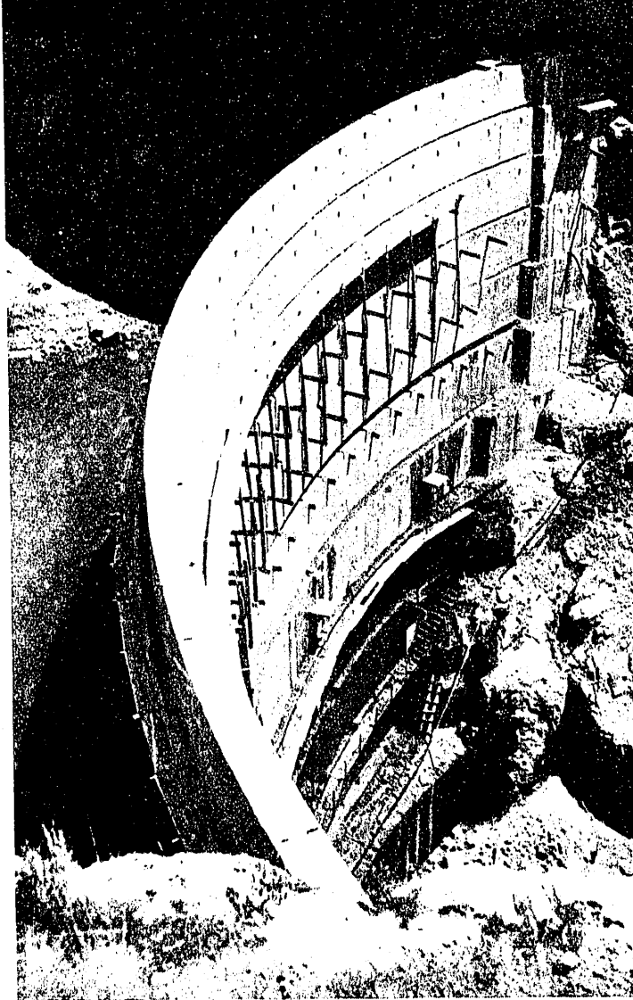
Presas de anillos. (Peña Boeuf.)
