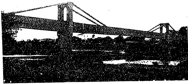
Acueducto de Fanjul, con tirantes pretensados. (L. Torroja.)
