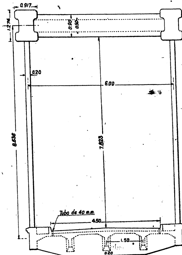
Corte transversal por la riostra.
