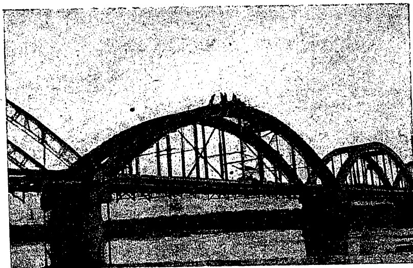
Construcción de un tramo sin andamiaje.
