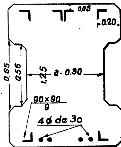
Secciones normales del arco.
