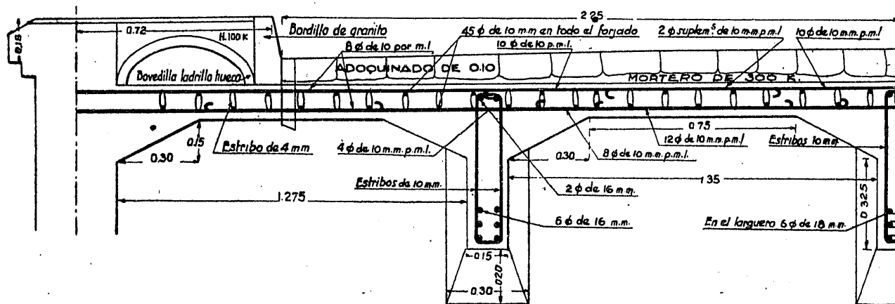
Forjados, largueros y tirantes. Semisección transversal por el centro de un larguero.
