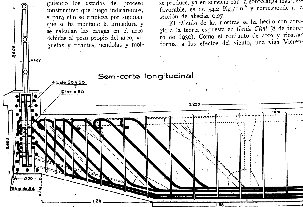
Sección del tirante y de la vigueta.
