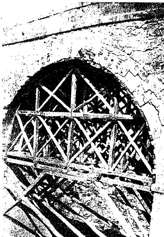
Fot. 2.ª Puente de las Viñas, en la misma carretera, con la sillería rota, que ha sido preciso apuntalar
