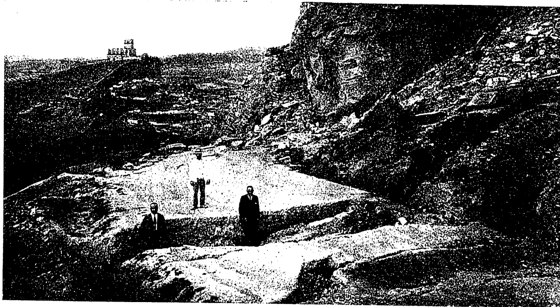
Fot. 4.ª Situación en que se halla el kilómetro 1 de la carretera de Montefrío a Tocón a causa del corrimiento ocurrido en abril de 1924
