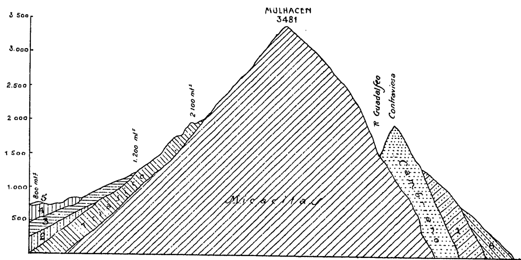
Fig. 8.ª Corte probable de Sierra Nevada tomado de Bertrand y Kilian 1, Numulítico; 2, Helvético; 3, Tortoniense y Salmático; 4, Yeso; 5, Caliza lacustre; 6, Plioceno marino
