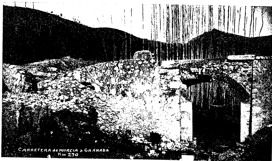
Fot. 5.ª Corrimiento del muro de acompañamiento de aguas abajo de un pontón sobre el río Darro en el kilómetro 270 de la carretera de Murcia a Granada
