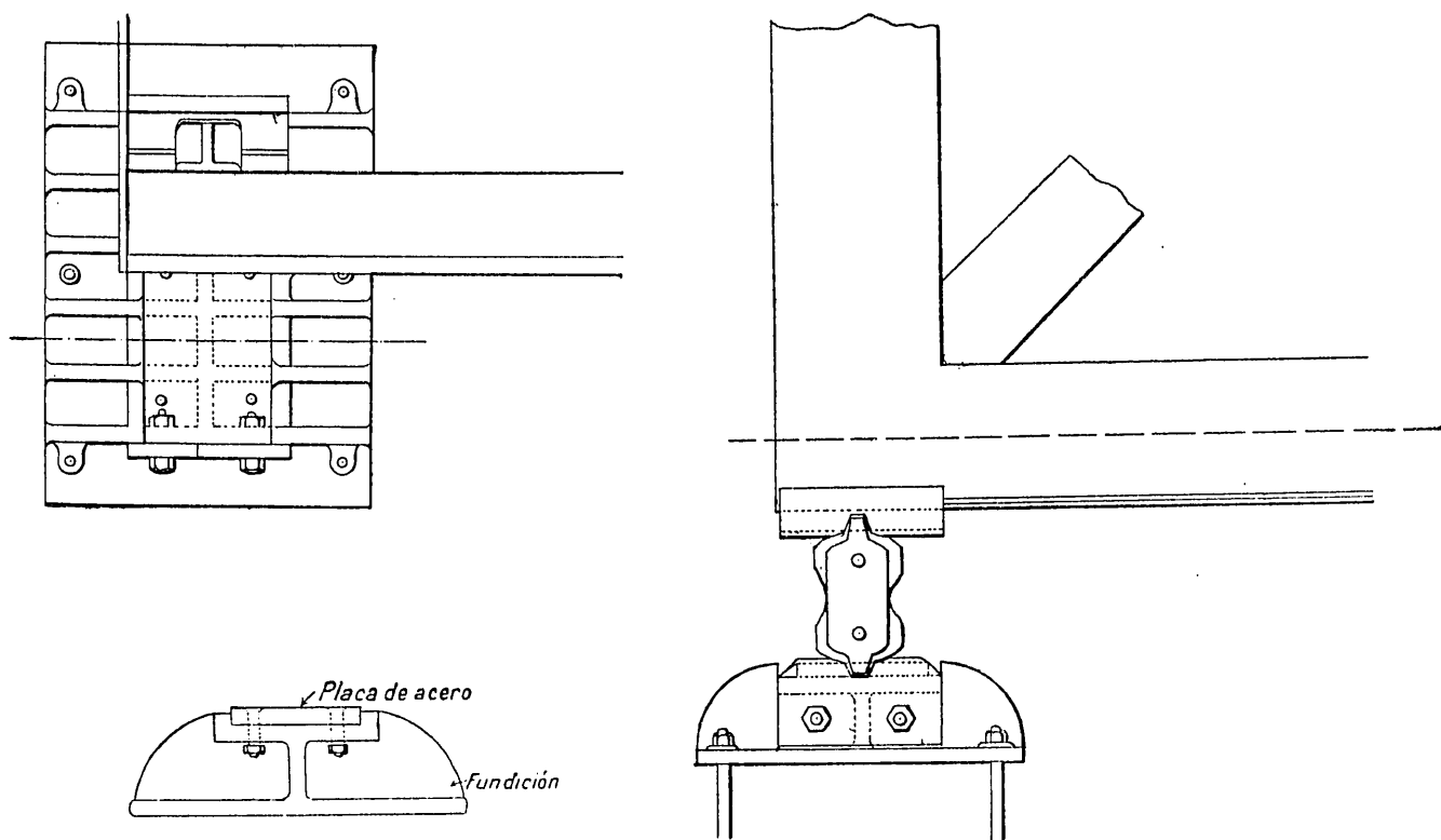
Apoyo en los estribos.
