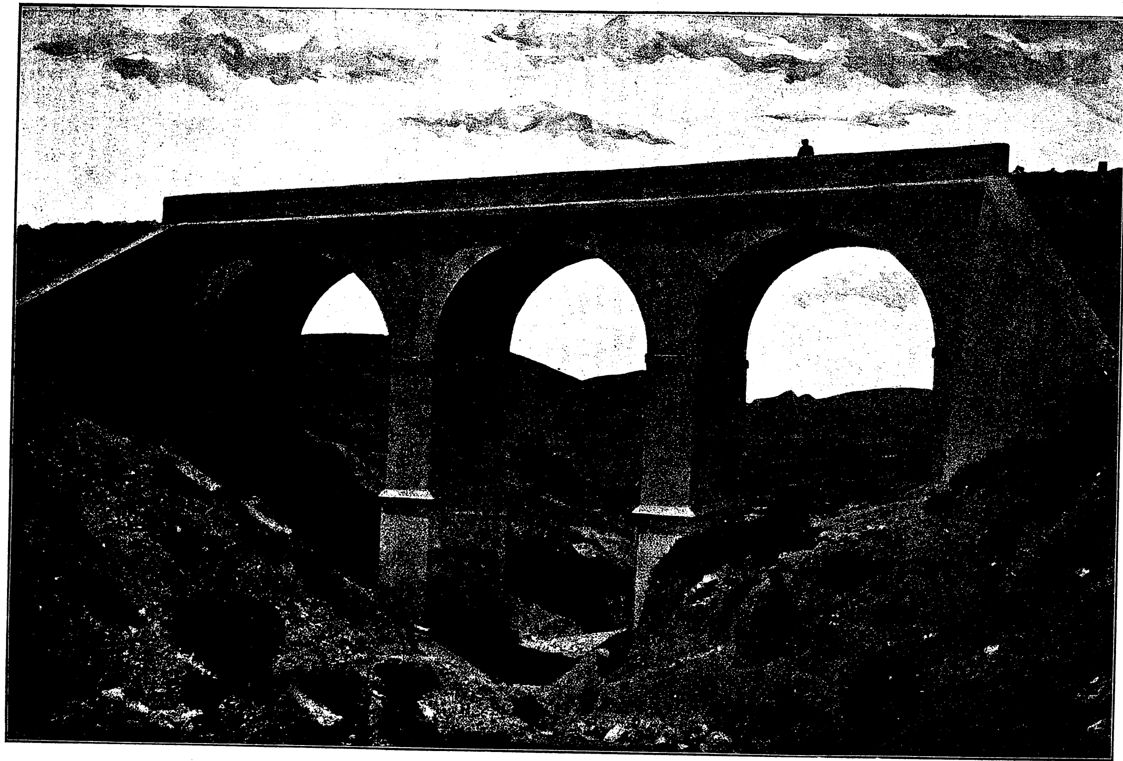
Viaducto de Saganta (Huesca).—Carretera de Güell á Binefar.
