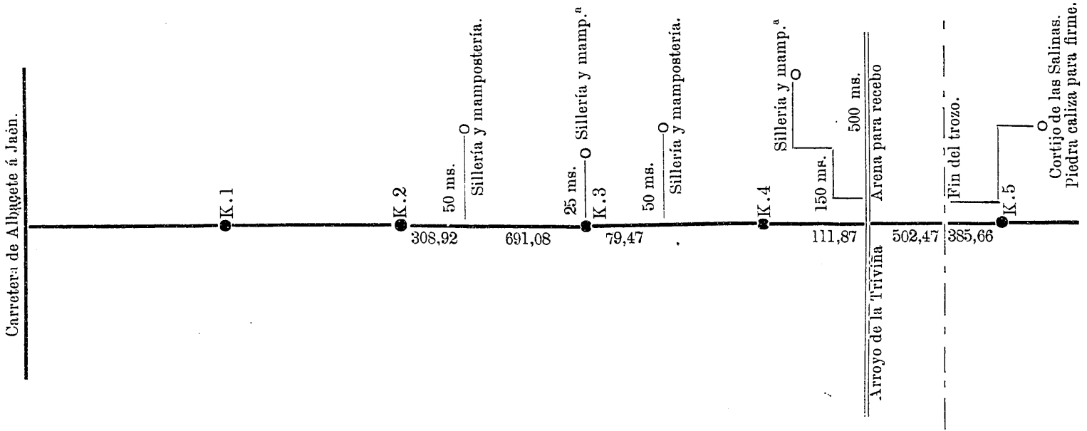
RELACION GRÁFICA DE CANTERAS
