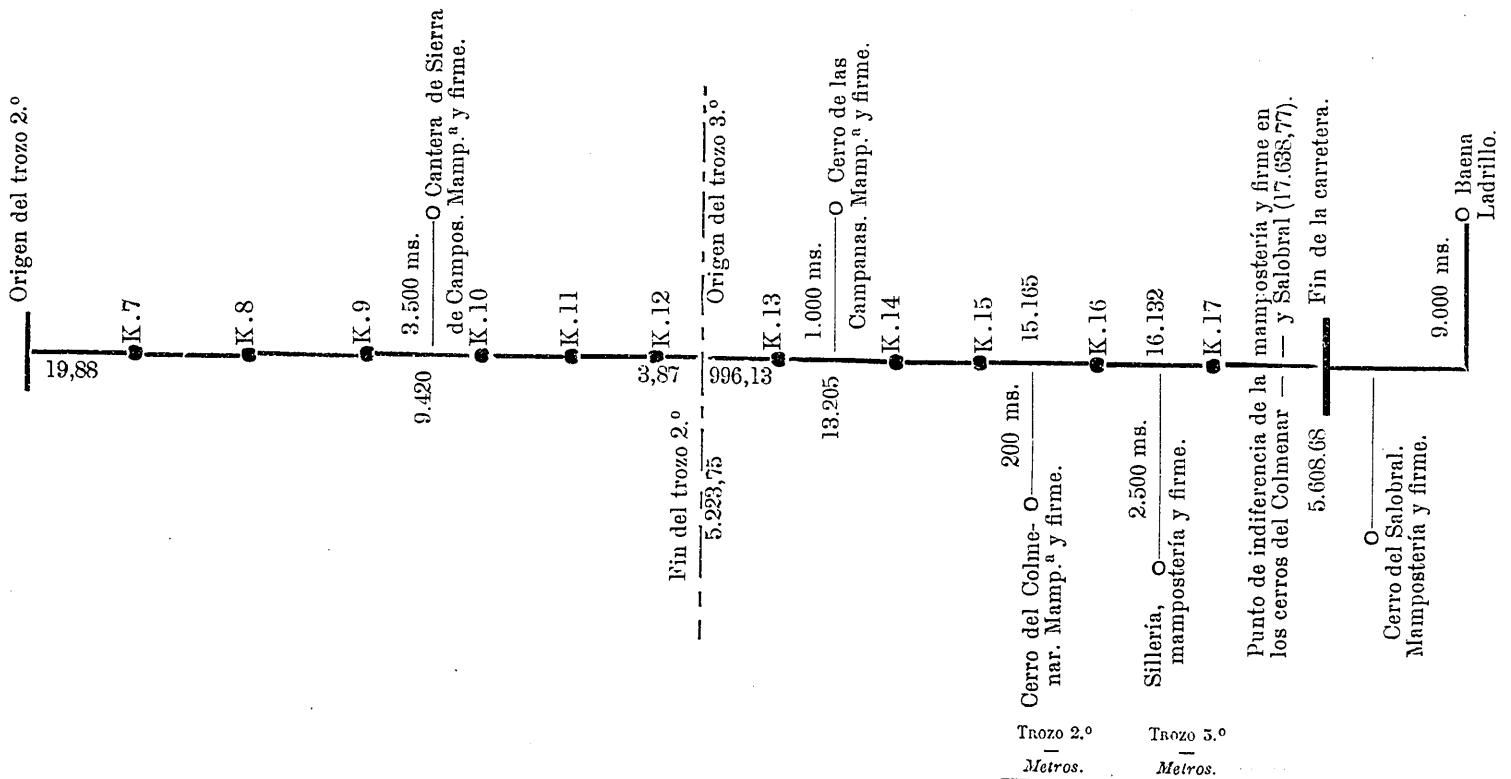
RELACION GRÁFICA DE CANTERAS
