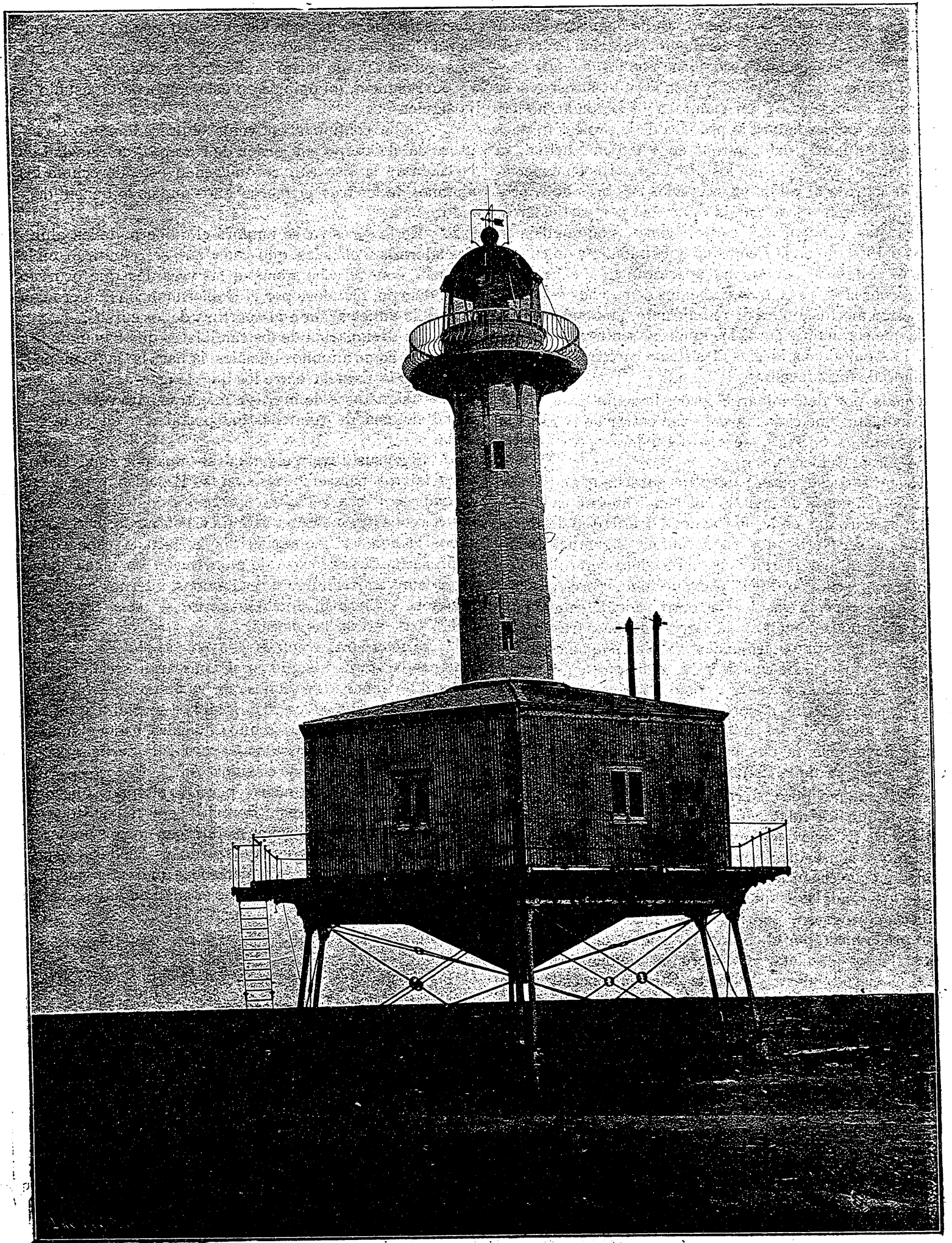
Faro de tercer orden de la Punta de la Baña (provincia de Tarragona).
