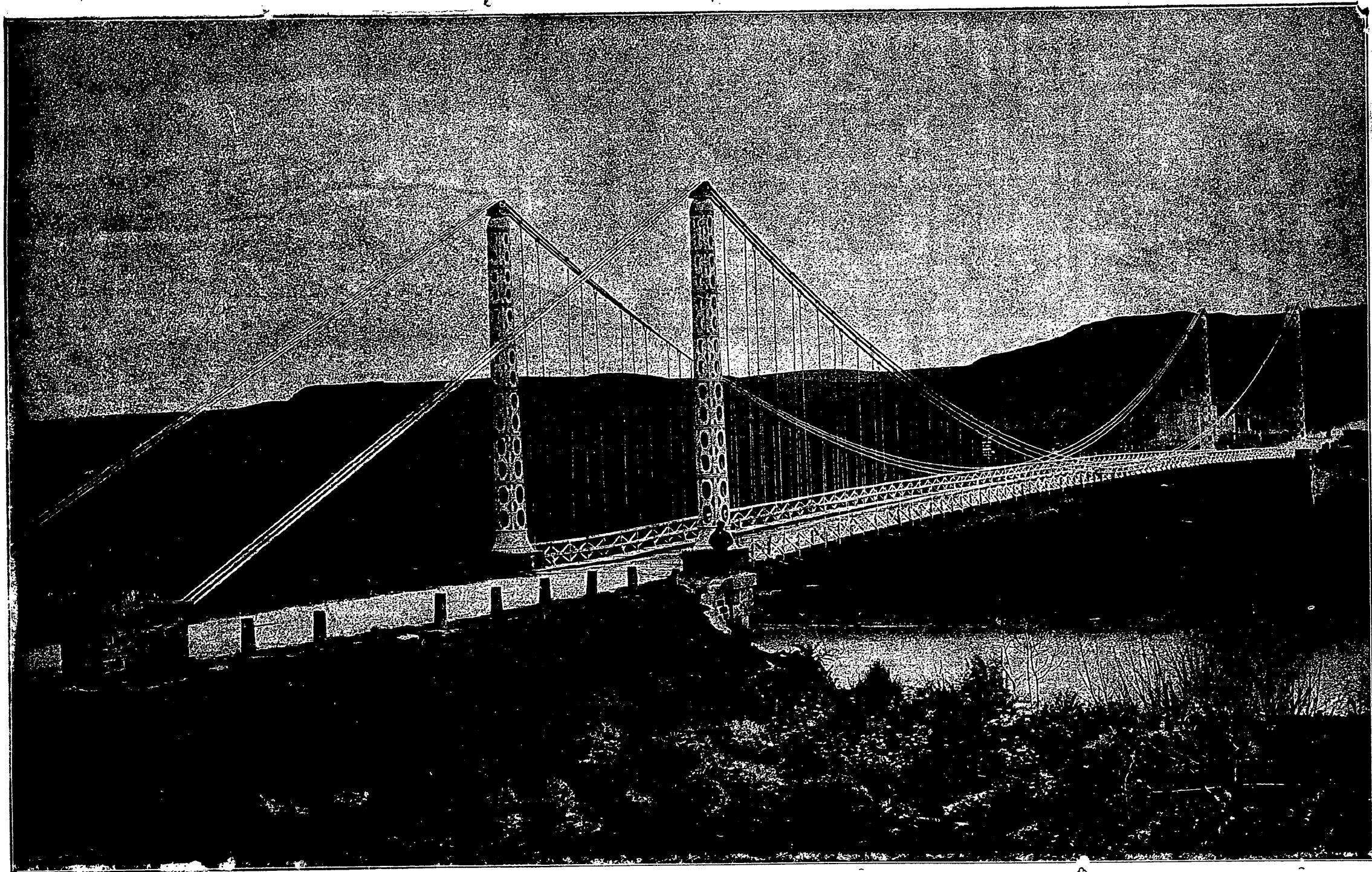
Puente de Menjíbar (108,50 metros de luz).—Carretera de Bailén á Málaga (Jaén).
