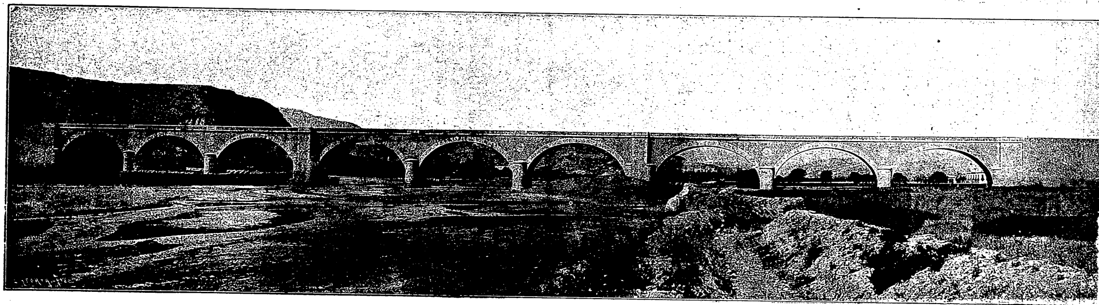
Puente sobre el río Andarax.—Carretera de Puerto-Lumbreras á Almería (Almería).
