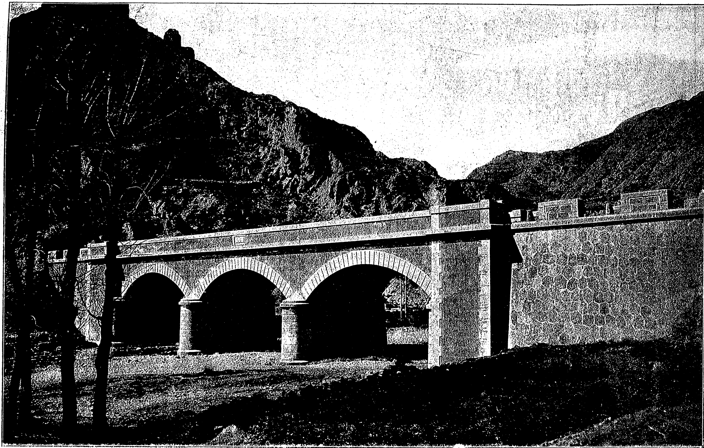
Puente sobre el río Llobregós.—Carretera de Folqué á Jorba (Barcelona).
