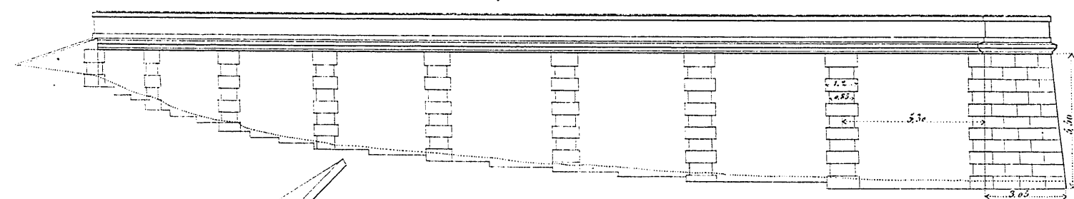
F. o 3. Proyeccion vertical de un estribo.
