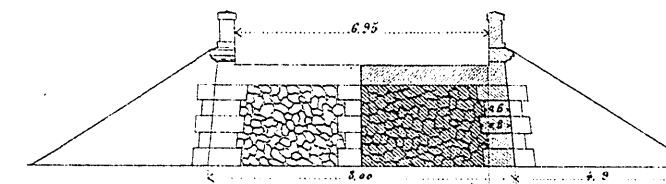
F. o 12. F. o 13. Proyeccion longitud. de un semi-estribo. Seccion longitudinal de id.
