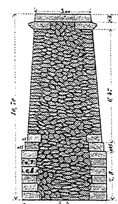
F. o 9. Seccion transversal.
