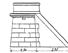
F. o 11. Proyeccion vertical.
