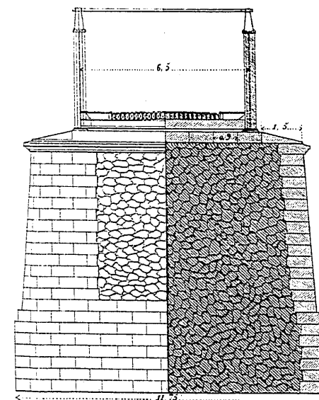
F. o 5. Proyeccion horizontal de una pila.
